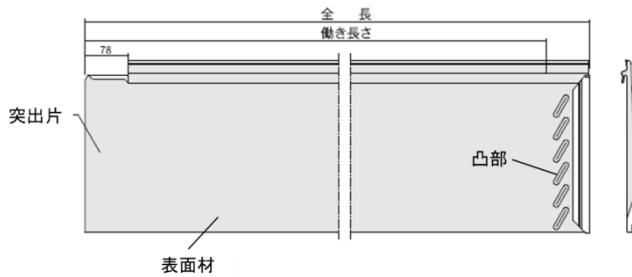
図1. 金属製横葺断熱屋根材製品図
